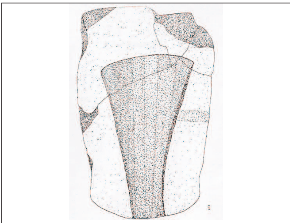
(Foto-3). Molde cerámico para la fabricación de hachas de bronce hallado en Almendralejo.
